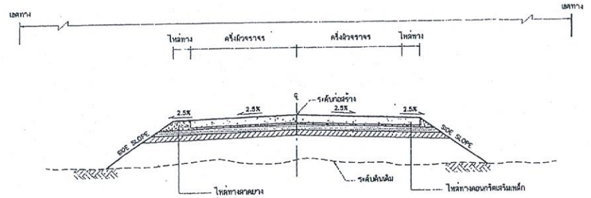
รูปตัดตามขวางแสดงดินถม
