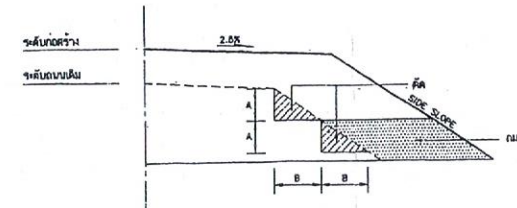
รูปตัดการก่อสร้างลาดชันทาง
