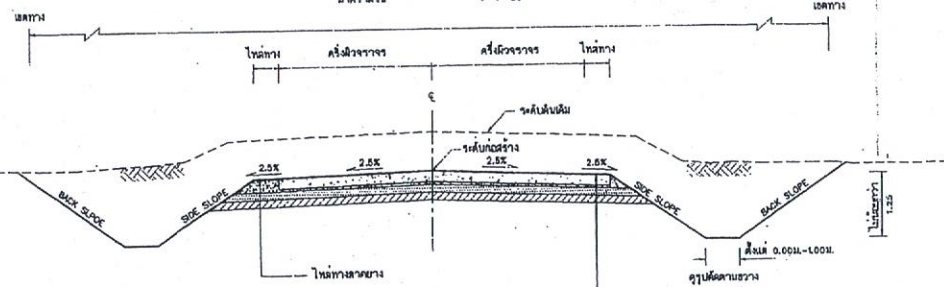
รูปตัดตามขวางแสดงดินหัด
